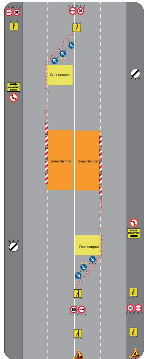
Exemple de périmètre de travaux
